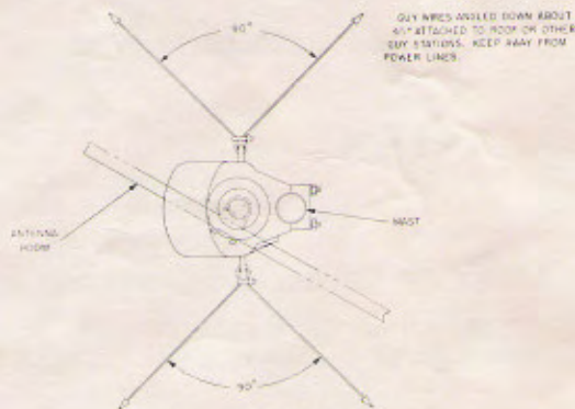
Fig. 2 — GUY WIRES
